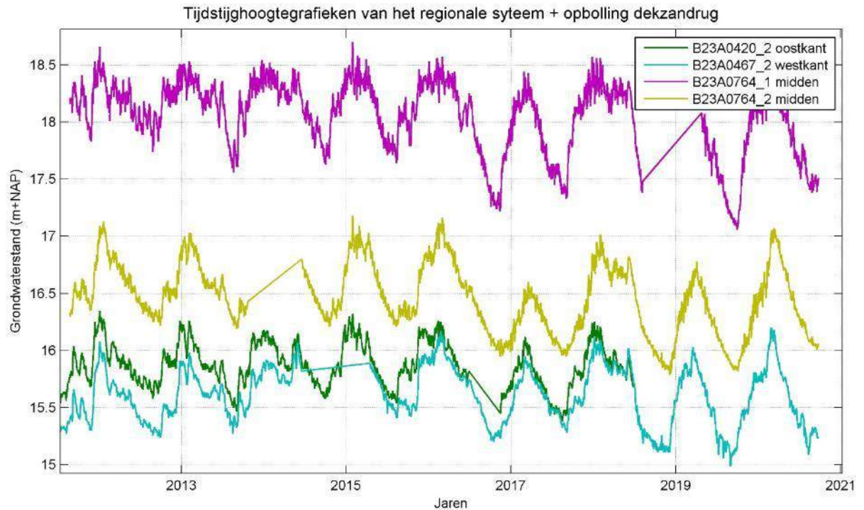
Figuur 5.5. Tijdstijghoogtegrafieken van 3 peilbuizen in het zandpakket onder de keileem, en één filter in de dekzandrug boven de keileem (paars).
